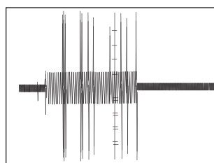
Startförlopp konventionell glimtändare
